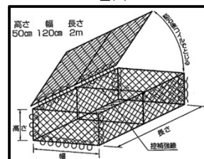
ふとん籠詳細図
