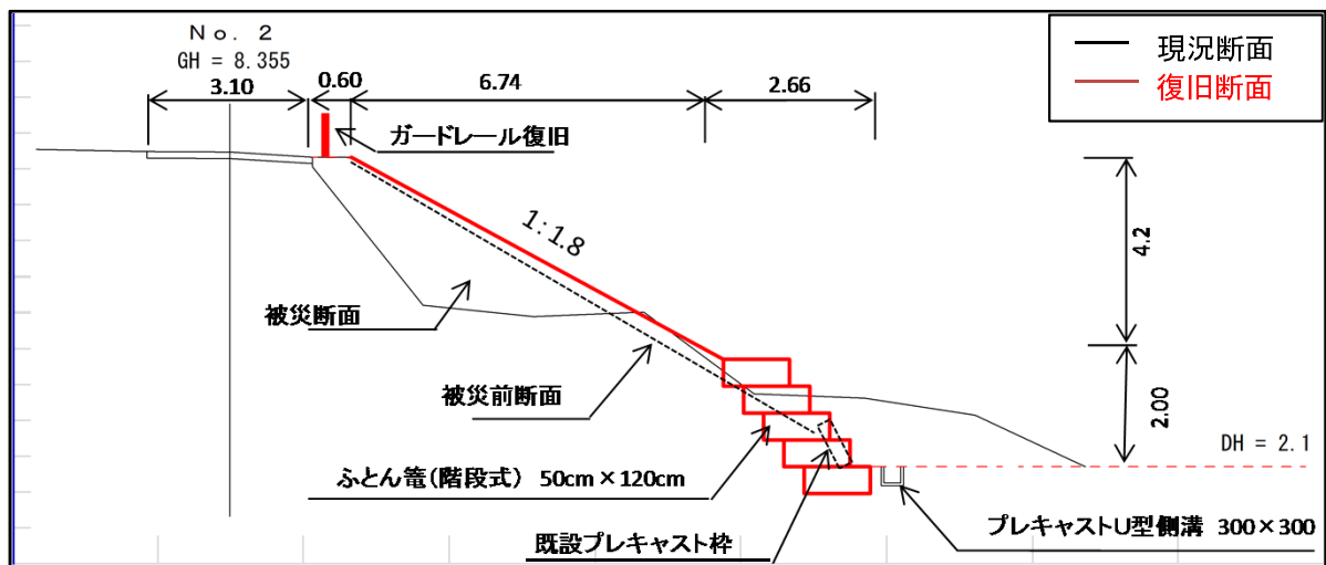
ふとん籠詳細図
