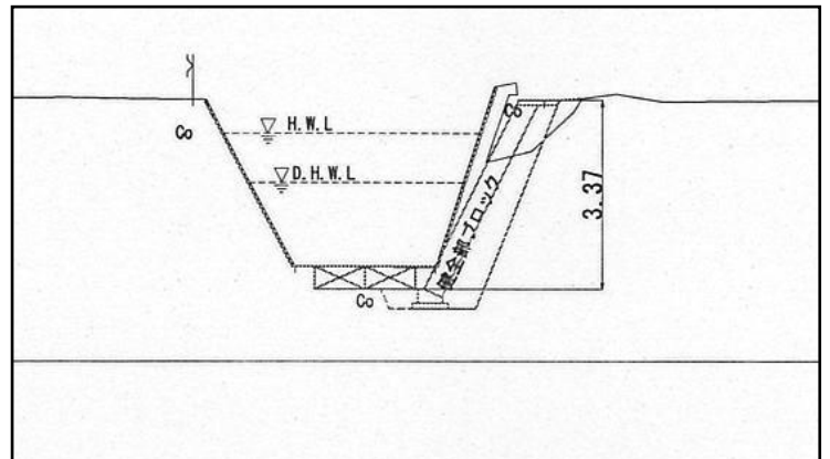
横断図
