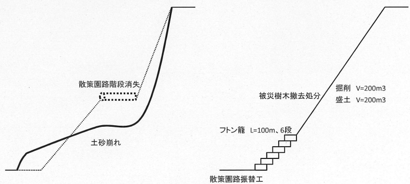
【横断図②】 ・被災状況
