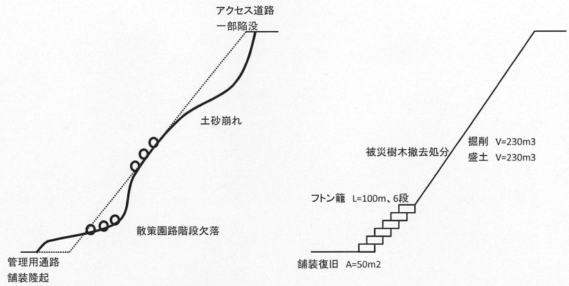
【横断図②】 ・被災状況
