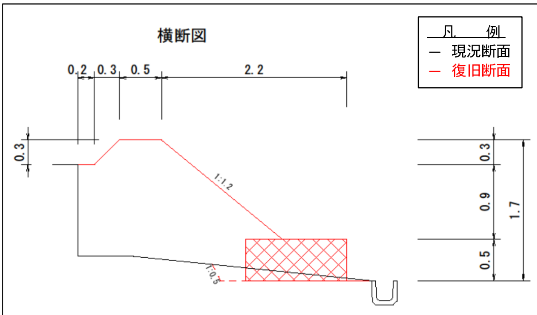
標準横断面図(復旧予定図)
