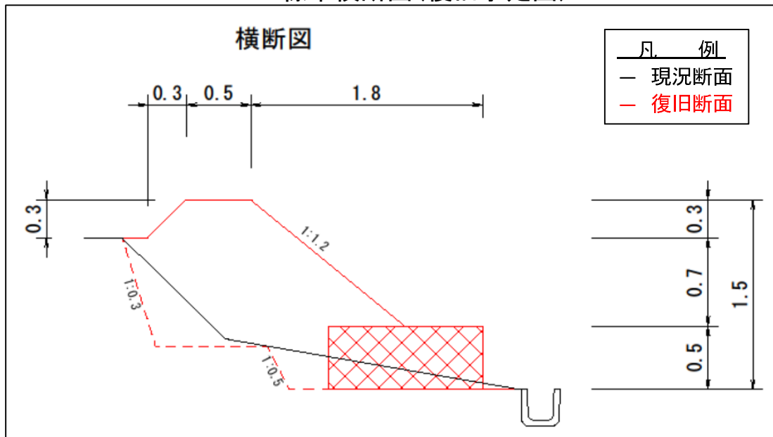
標準横断面図(復旧予定図)
