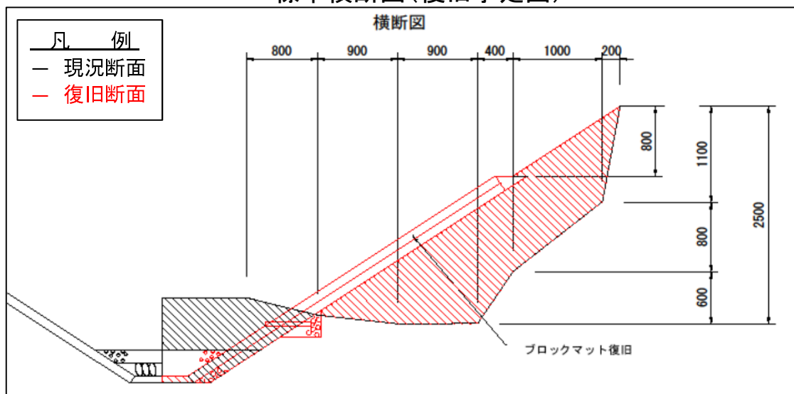
ブロックマット詳細図
