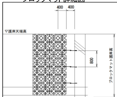
ブロックマット詳細図
