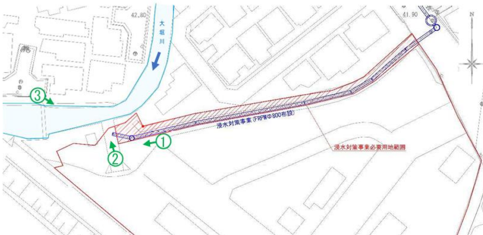
平面図
