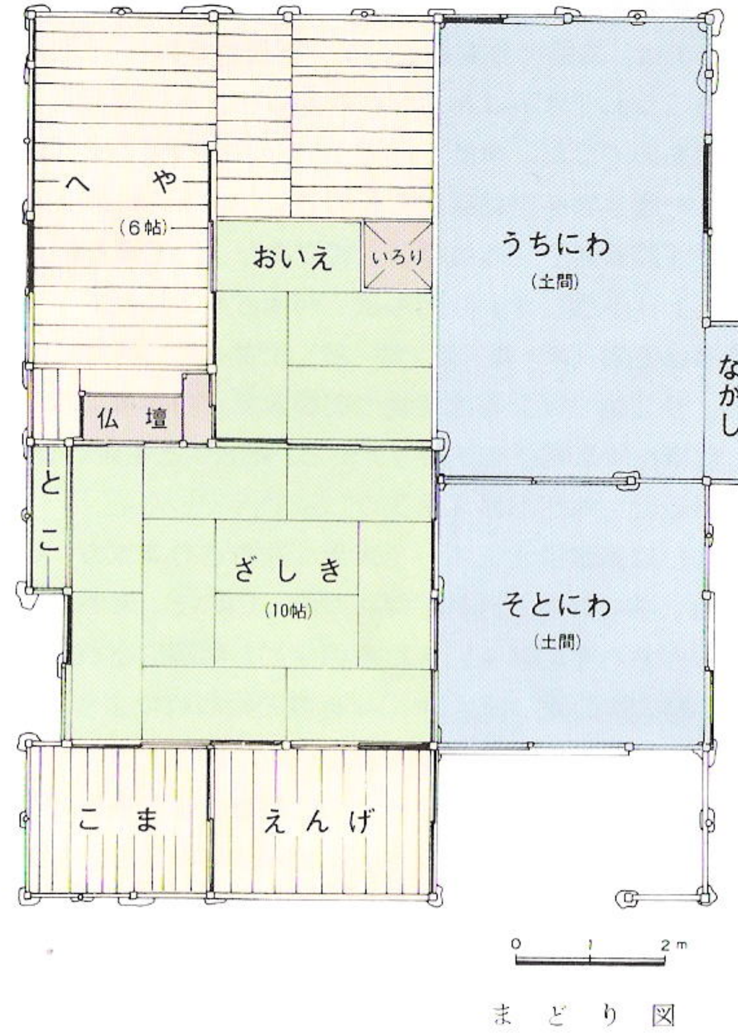
宝塚市立歴史民俗資料館旧東家住宅平面図
