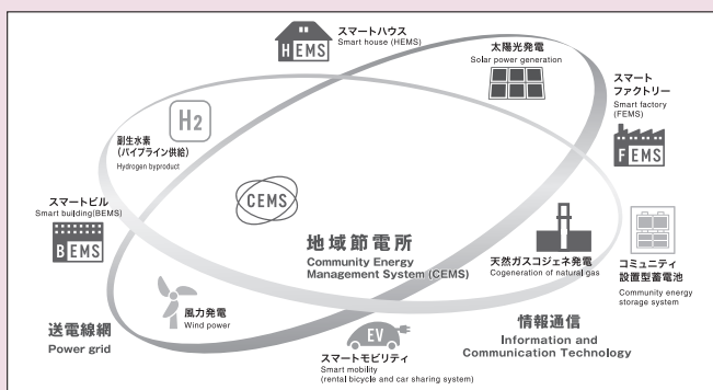
CEMSのイメージ図(提供:北九州市役所)
