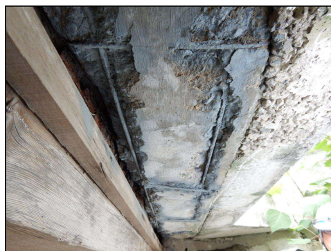
主桁に剥離・鉄筋露出が見られます
