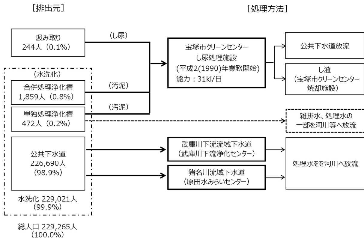
生活排水処理システムの概要（令和 5（2023）年度）
