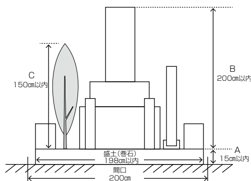
普通墓所（長尾山霊園）墓石建立基準図（正面） （第1区～23区 間口2m・奥行き2mの場合）
