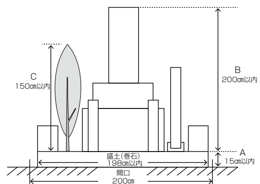
(例) 普通墓所（長尾山霊園）墓石建立基準図（正面） （第1区～23区 間口2m・奥行き2mの場合）
