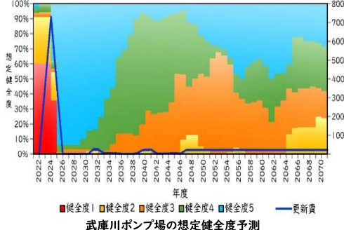
武庫川ポンプ場の想定健全度予測
