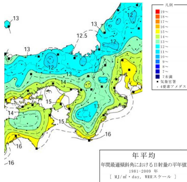
図1-2 年間最適傾斜角における日射量の平年値
