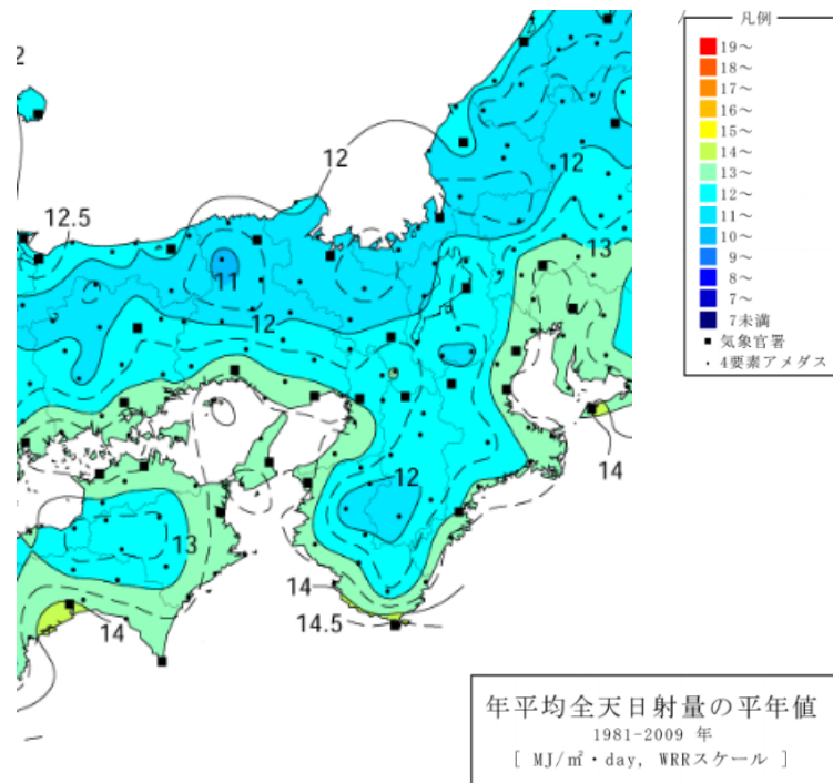
図1-1 年平均全日射量の平年値
