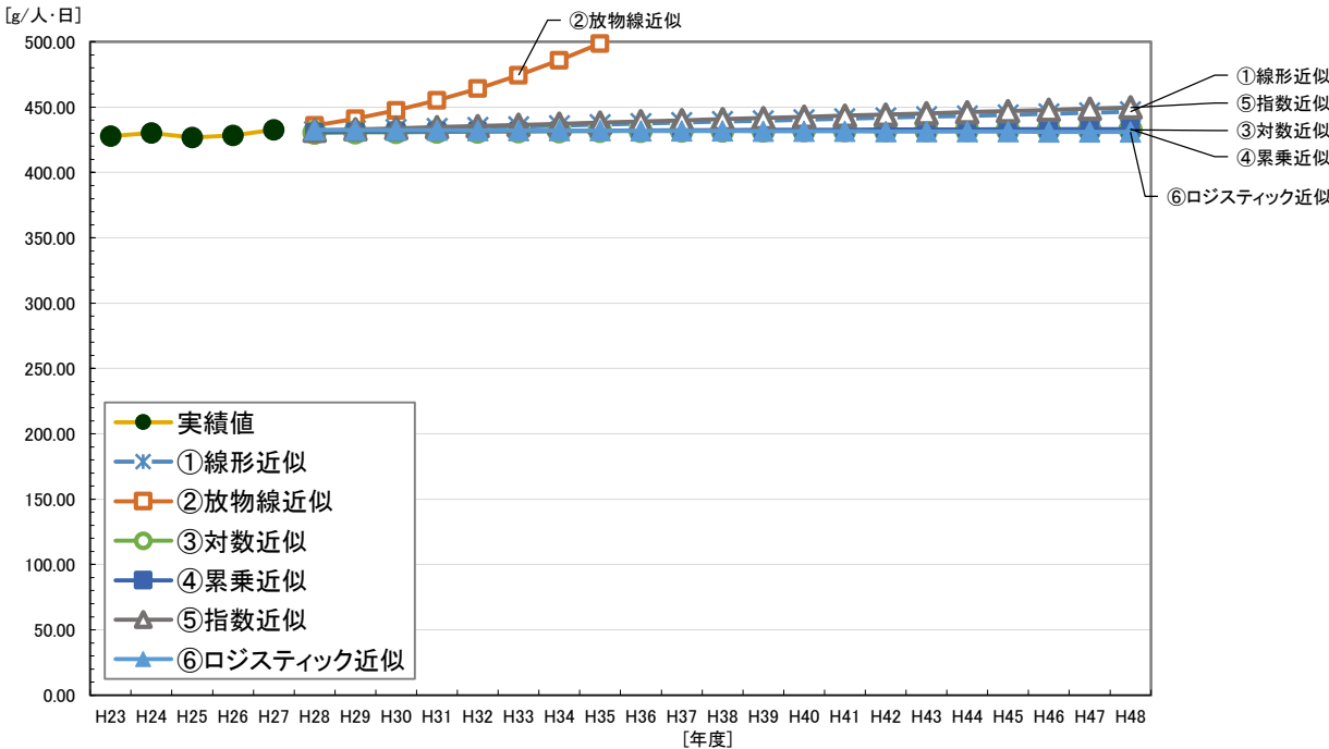
図 燃やすごみ(家庭系)の発生原単位の推移及び各推計式による推計結果
