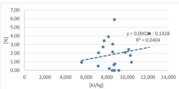
図 低位発熱量と繊維類の散布図
