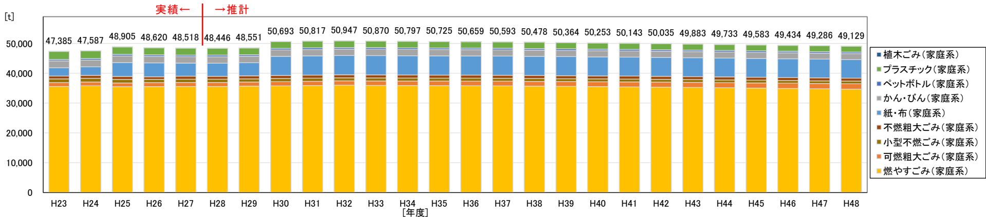
図 家庭系ごみ量の推計結果
