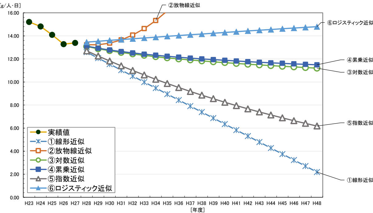
図 小型不燃ごみ(家庭系)の発生原単位の推移及び各推計式による推計結果
