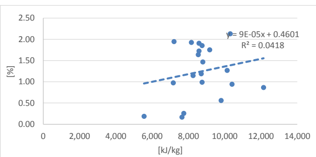
図 低位発熱量と 5mm のふるいを通過する物の散布図
