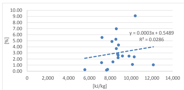
図 低位発熱量と 5mm のふるいを通過しない物の散布図
