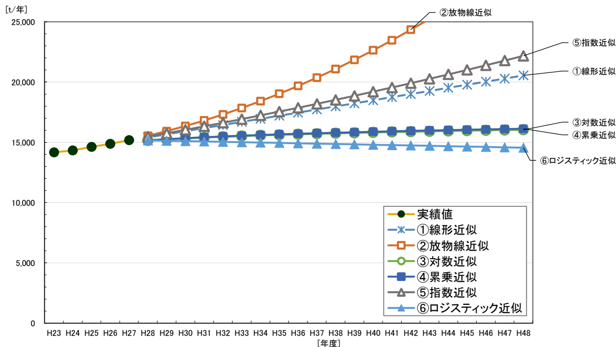
図 燃やすごみ(事業系)の発生量の推移及び各推計式による推計結果
