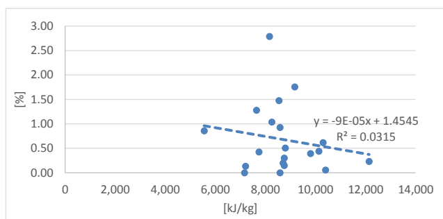
図 低位発熱量と金属類の散布図
