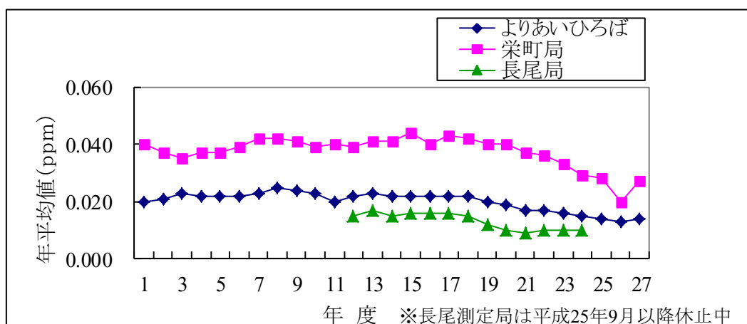
【図3】 二酸化窒素の年平均値
