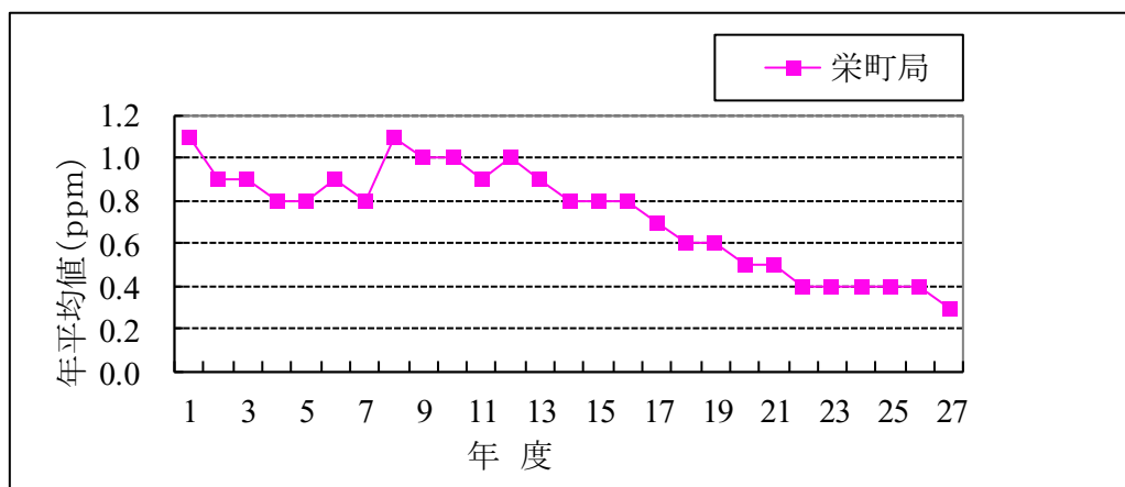
【図6】一酸化炭素の年平均値
