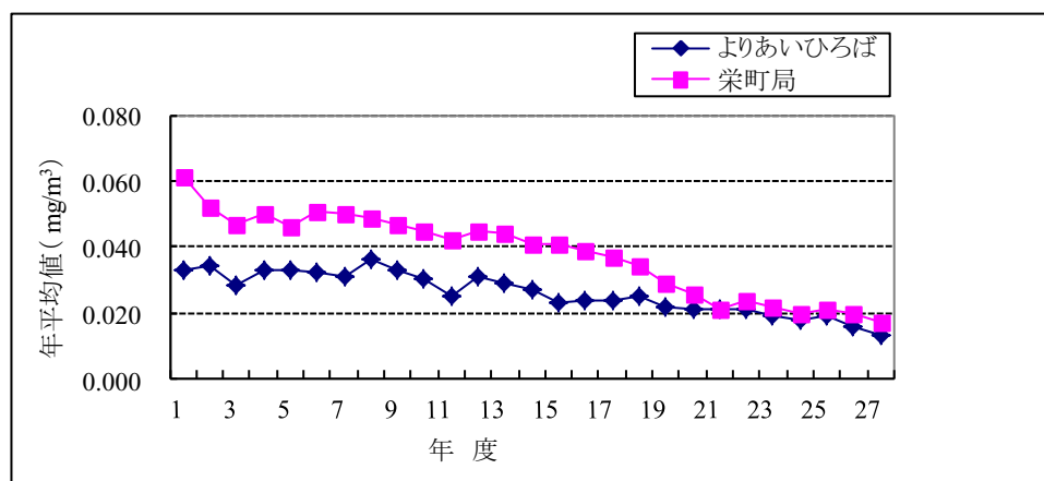
【図5】浮遊粒子状物質の年平均値
