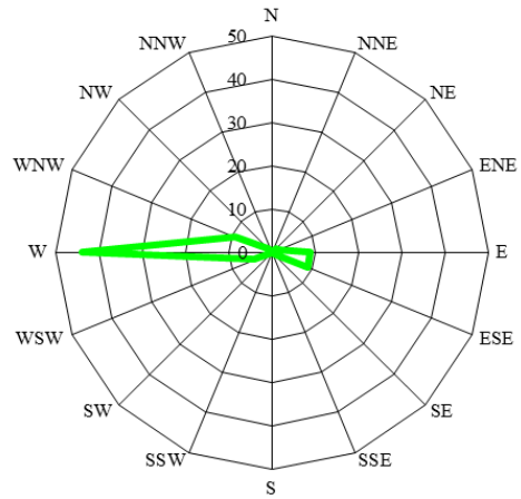
【図9】栄町測定局風況図
