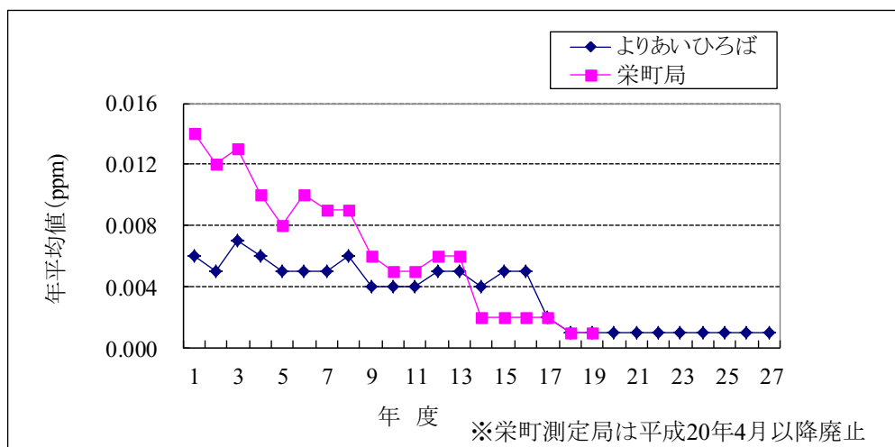
【図2】二酸化硫黄の年平均値
