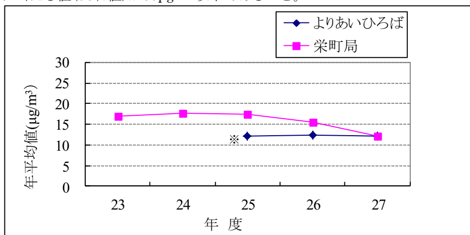
【図7】 PM 2.5 の年平均値
