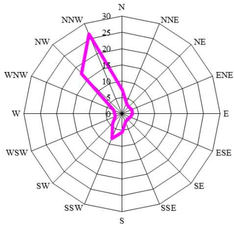
【図8】よりあいひろば風況図
