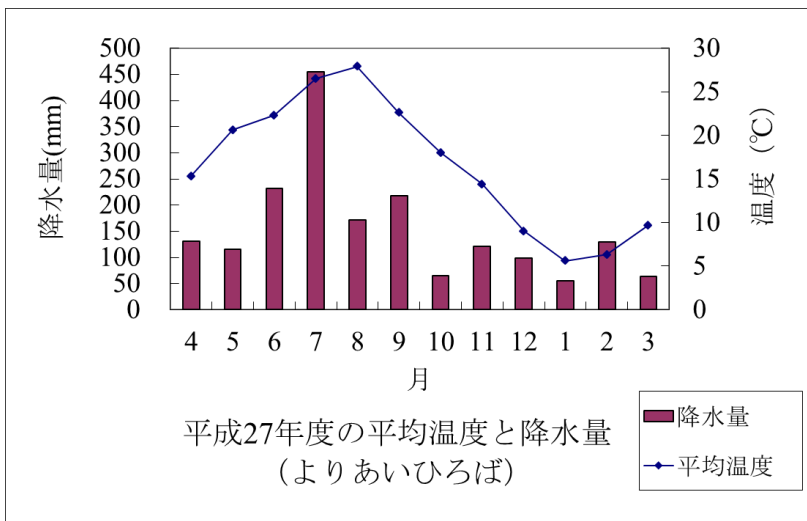
【図11】よりあいひろば気象
