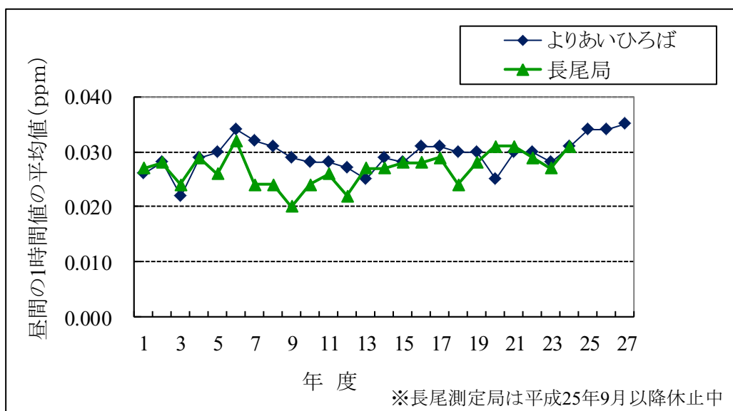
【図4】光化学オキシダントの年平均値
