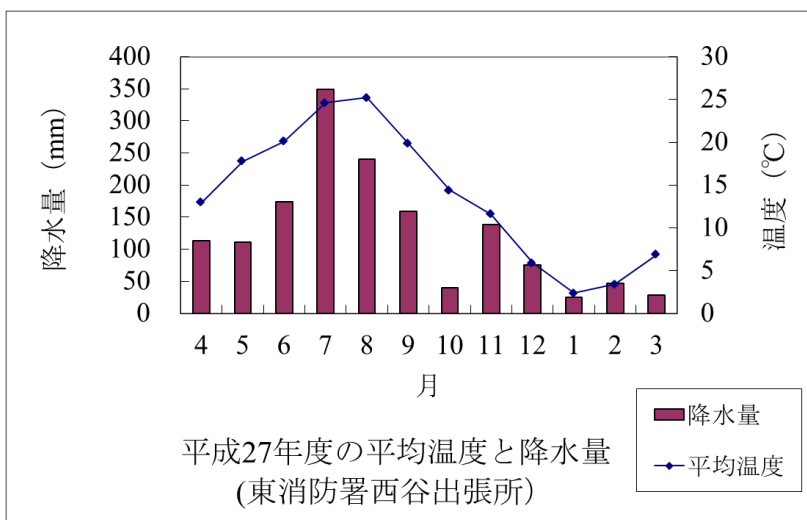
【図12】東消防署西谷出張所気象
