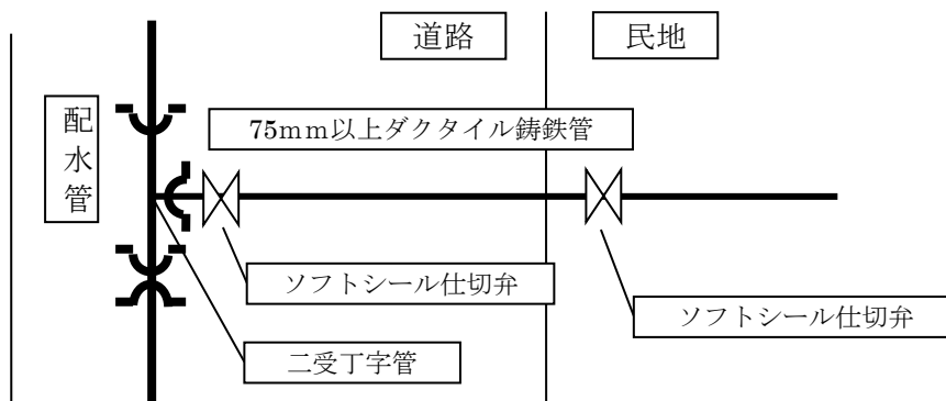
図 6 - 3 二受丁字管 75\text{mm} 以上の分岐方法
