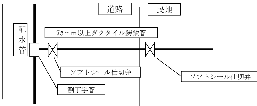
図 6 - 2 不断水割丁字管 75\text{mm} 以上の分岐方法
