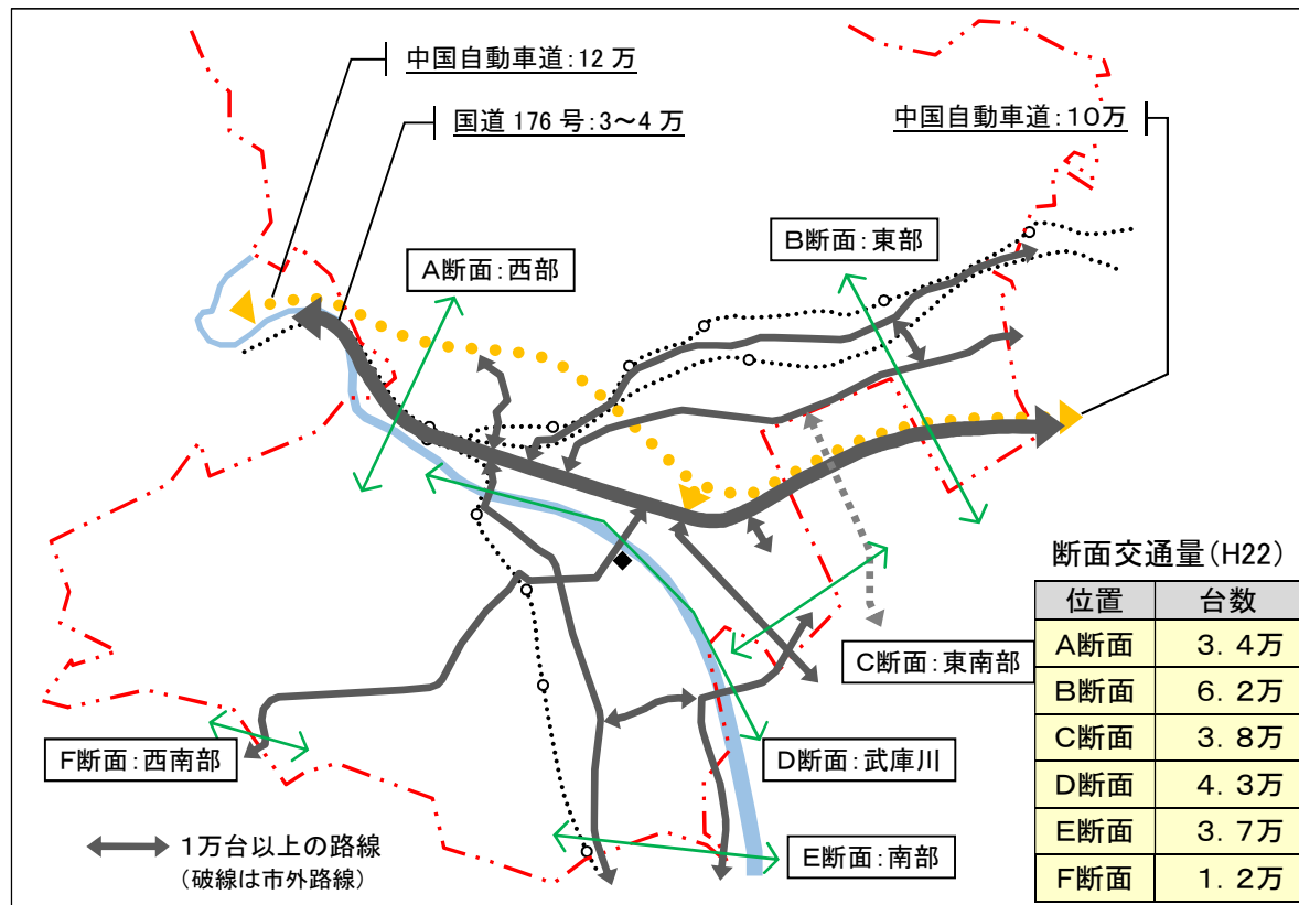
図：市と隣接する道路における現況交通量（平成 22 年(2010 年)交通センサス OD※より）
