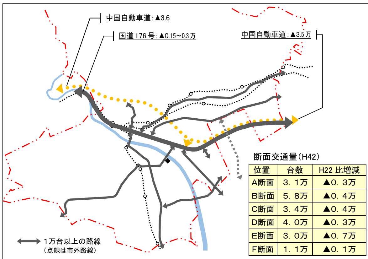
図：現道路網での交通量の将来見通し（将来 OD（平成 42 年(2030 年)）による配分手法による）
