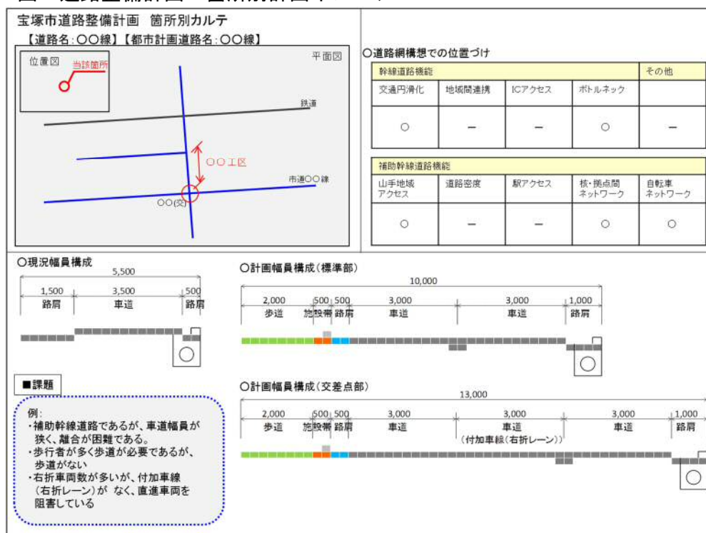
図：道路整備計画 箇所別計画イメージ
