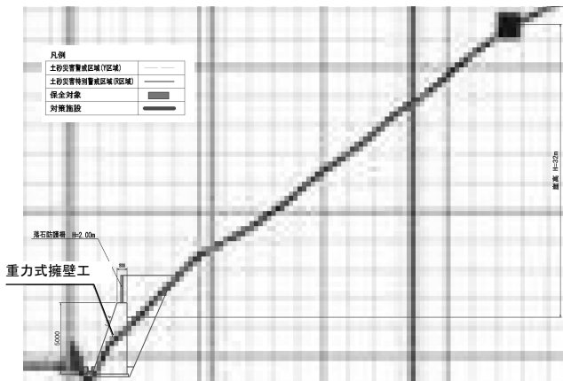
計画断面図（概略検討）
