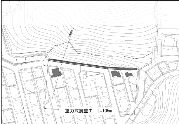
計画平面図（概略検討）
