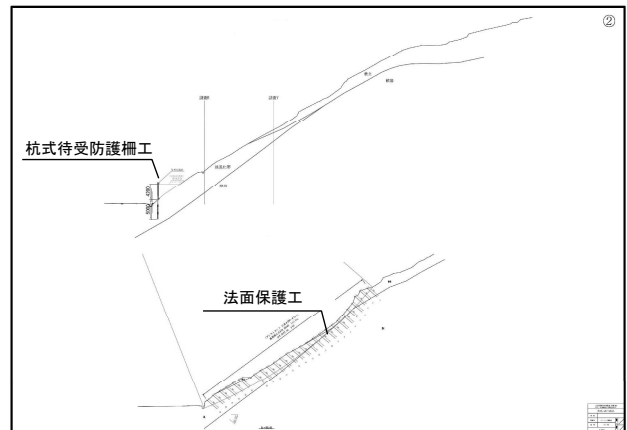
計画断面図（詳細設計）
