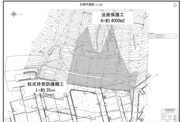
計画平面図（詳細設計）
