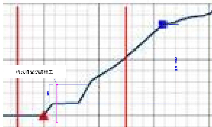
計画断面図
