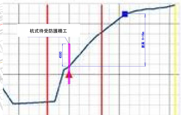
計画断面図（概略検討）
