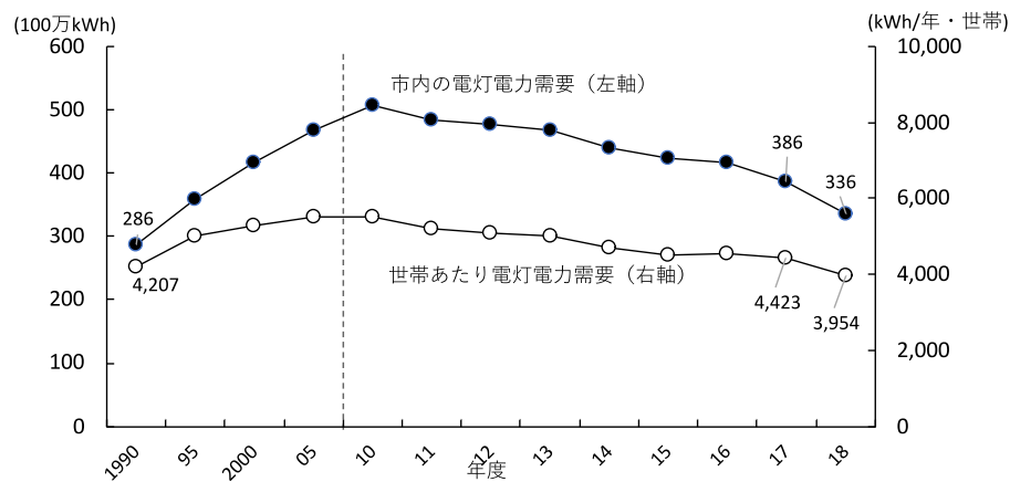
図 2-19 電灯電力需要の推移
