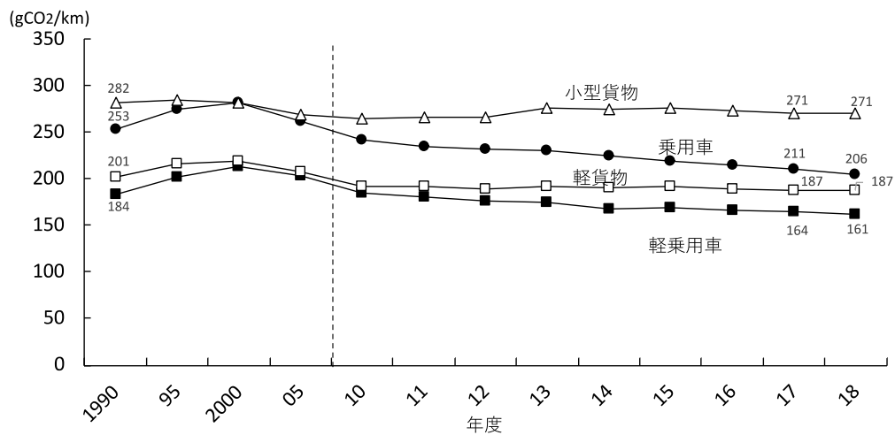
図 2-28 走行距離当たり CO 2 排出量の推移
