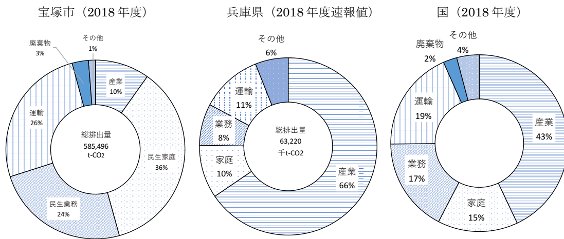
図 2-31 本市、国及び兵庫県の排出量内訳
