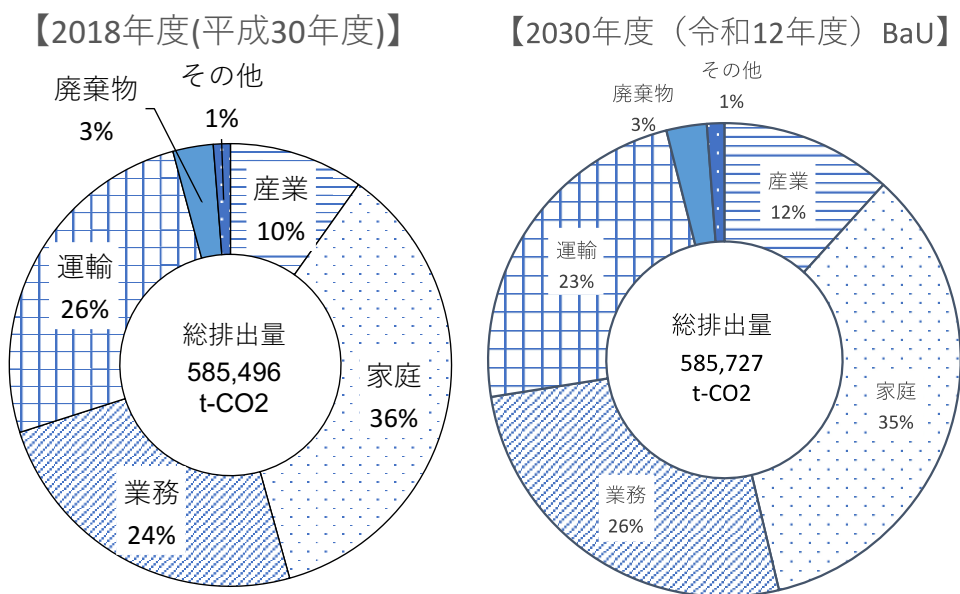
図 3-2 BaU 排出量推計結果（排出量内訳）
