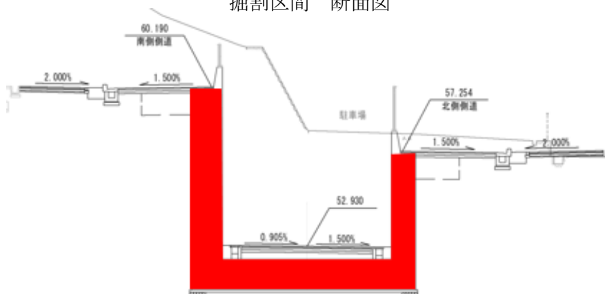
掘削区間 断面図
