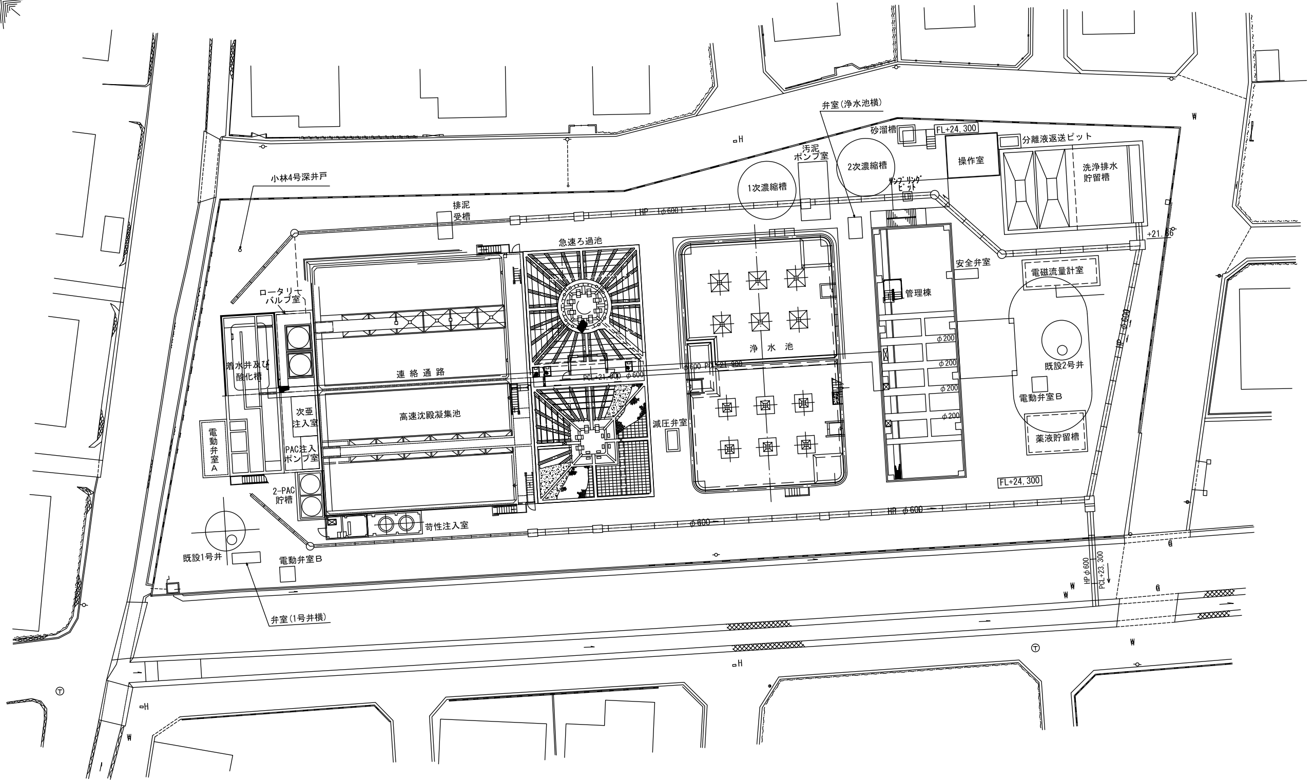
小林浄水場 一般平面図 S=1:200
