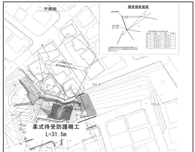
計画平面図（月見山2丁目）
