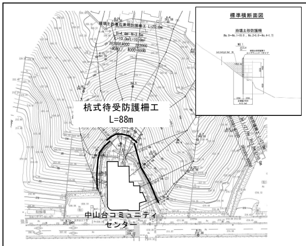
計画平面図（中山桜台5丁目）
