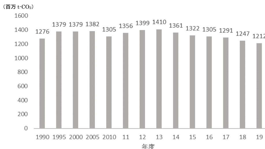
図 1-2 国内の温室効果ガス排出量の推移
