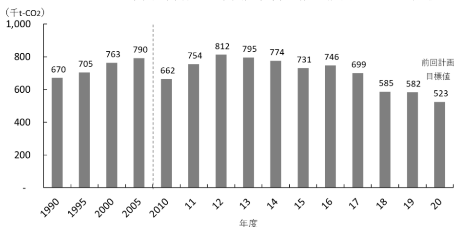
図 2-14 温室効果ガス総排出量の推移
