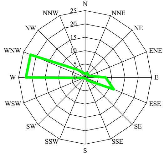
【図9】 栄町局風況図
