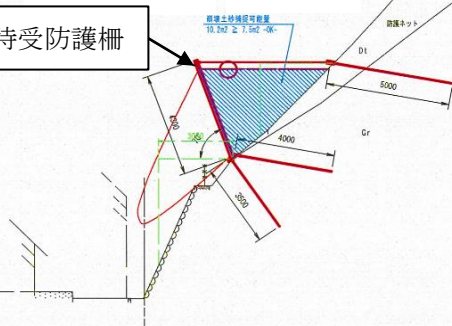
標準横断面
