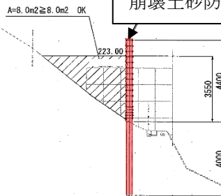
標準横断面
