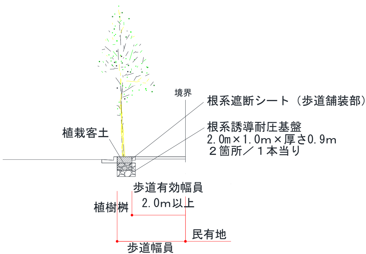
歩道横断方向耐圧基礎施工（案）断面図
