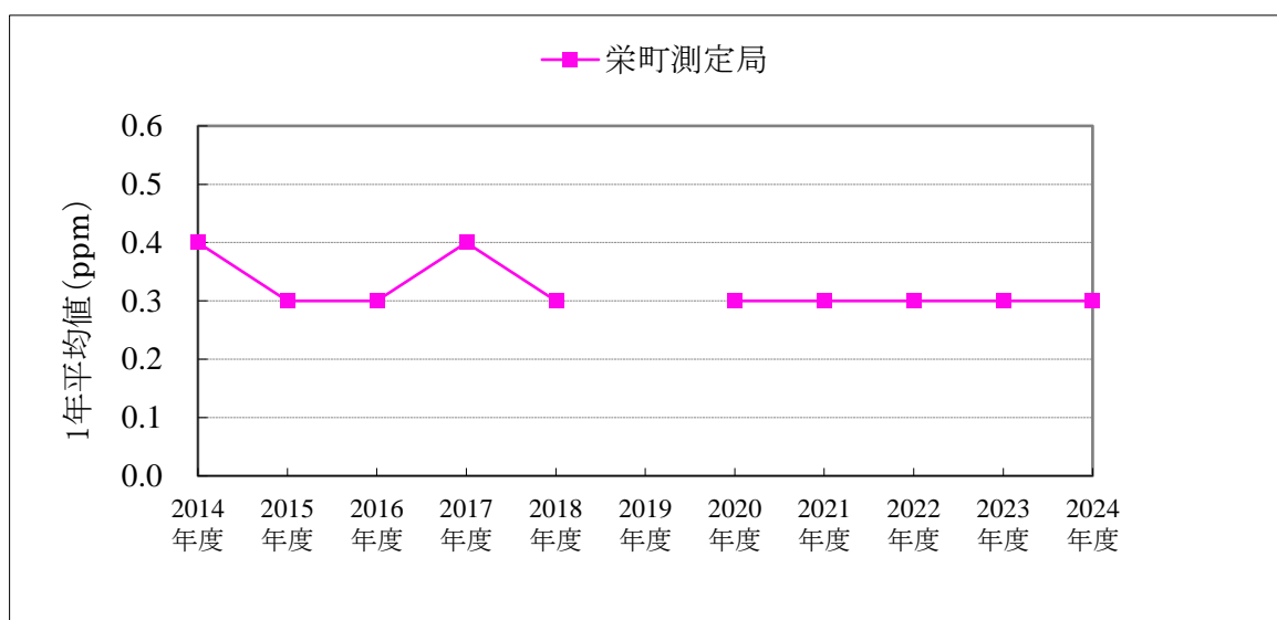
一酸化炭素の経年変化(1 年平均値)
