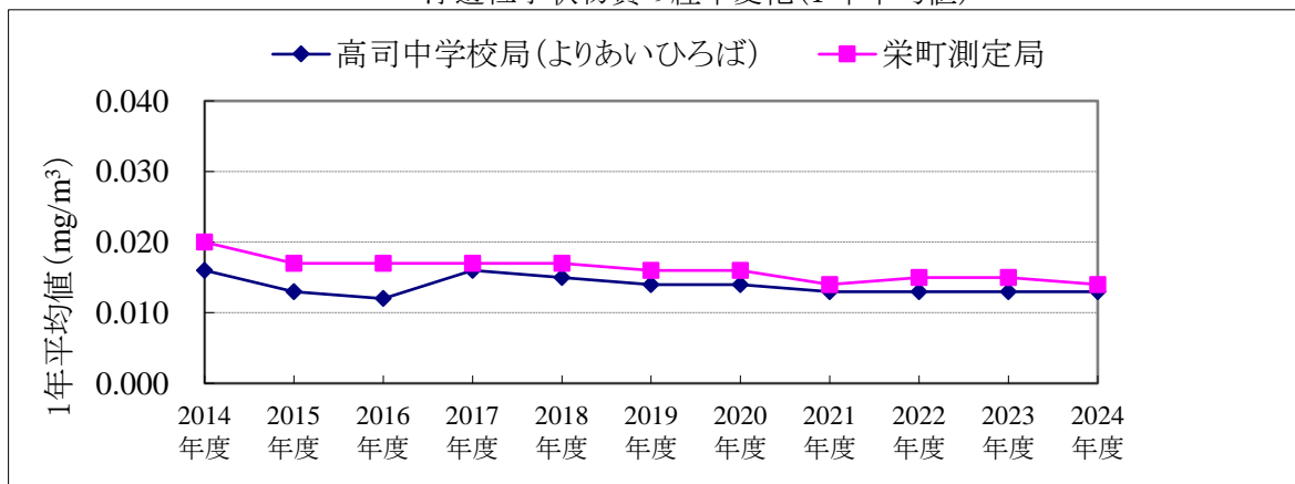
浮遊粒子状物質の経年変化(1年平均値)
