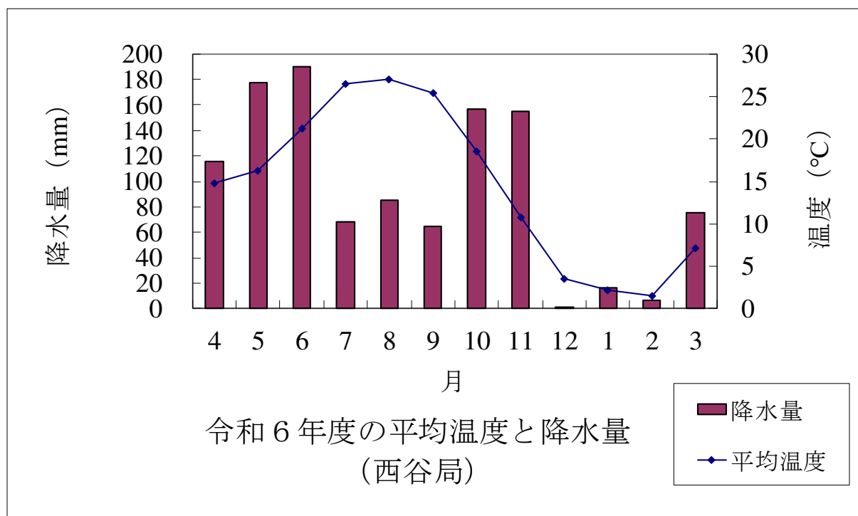
【図12】 西谷局 気象
