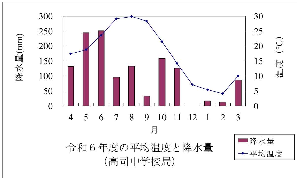
【図11】 高司中学校局 気象
