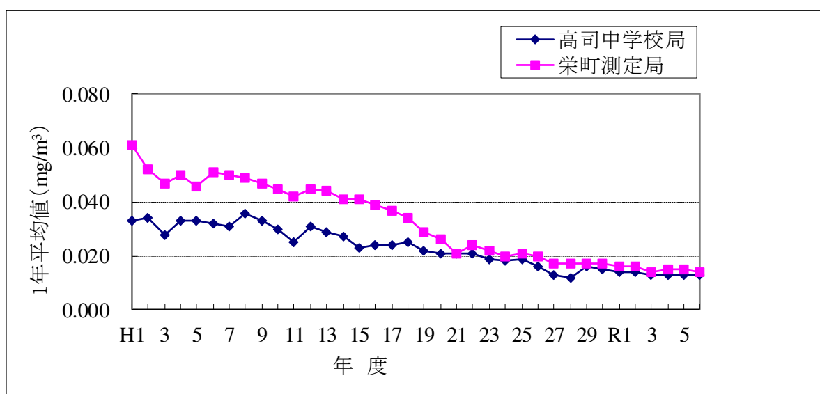
【図5】浮遊粒子状物質の1年平均値の推移
