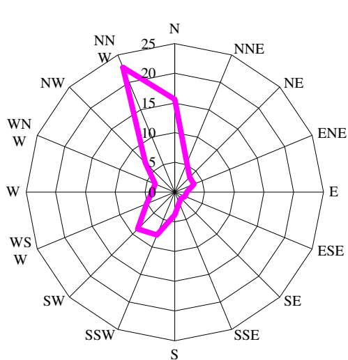
【図8】高司中学校局風況図
