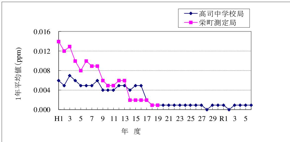
【図2】二酸化硫黄の1年平均値の推移
