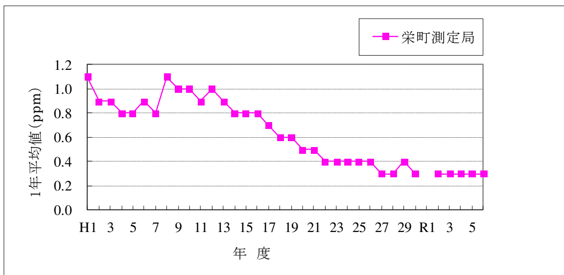
【図6】一酸化炭素の1年平均値の推移
