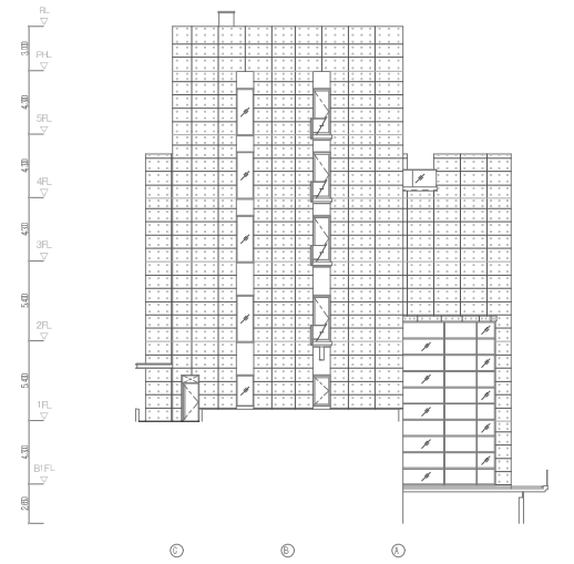
東立面図
