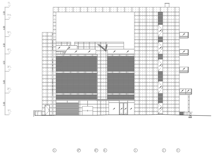
南立面図
