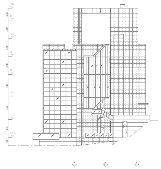
西立面図
