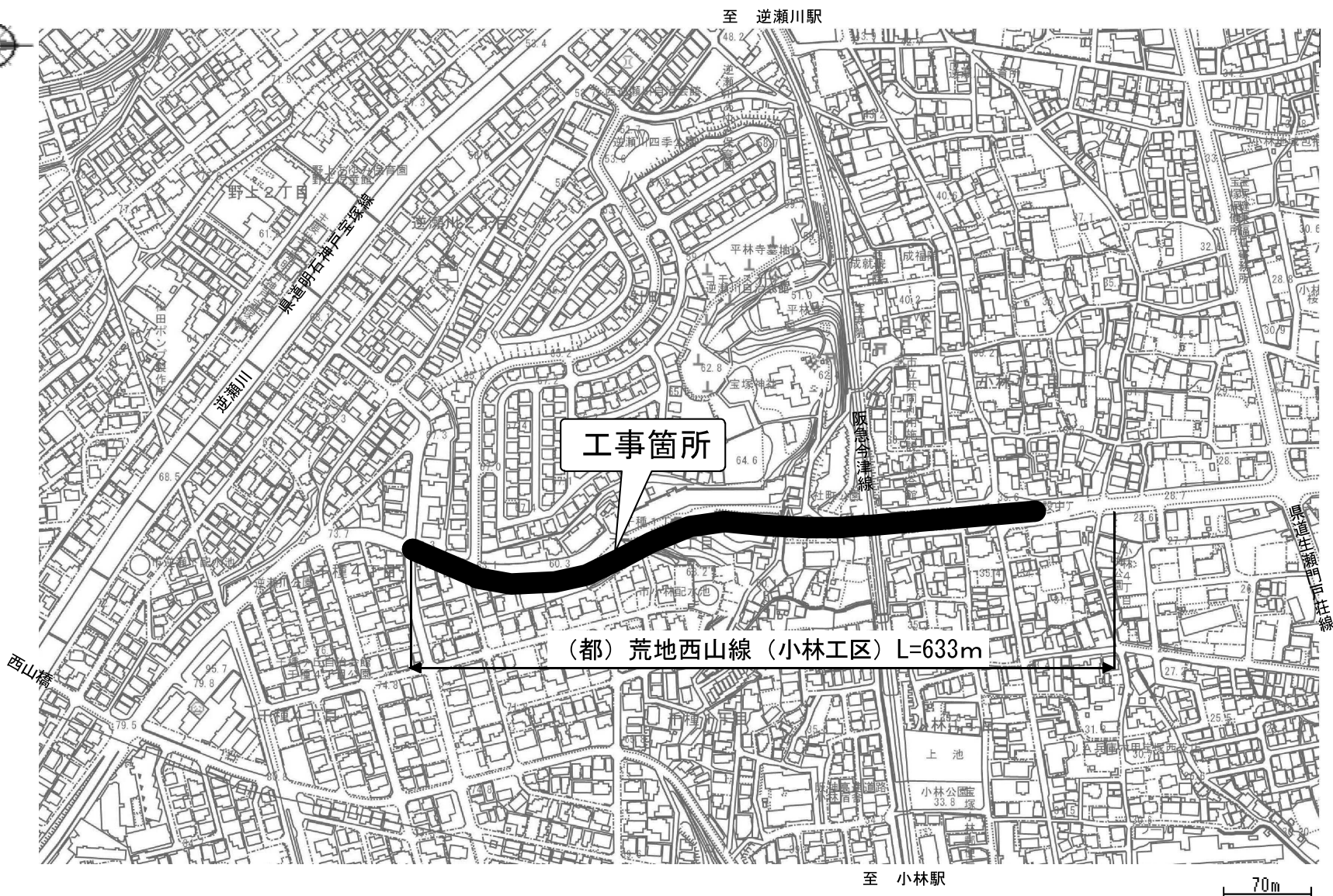
付近見取図 S = 1 : 5,000
